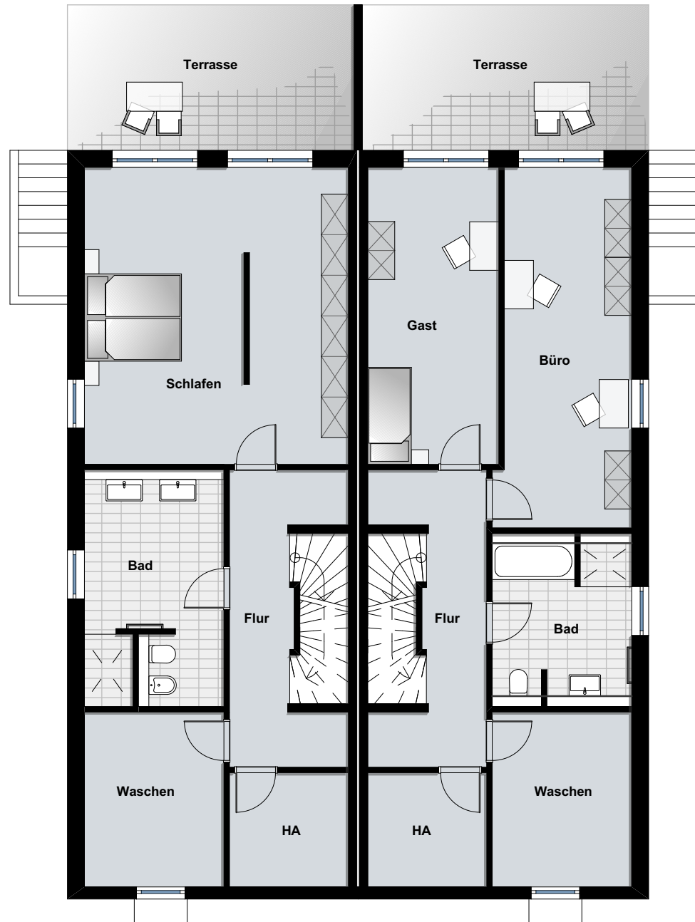
Untergeschoss HS 1 + 3
